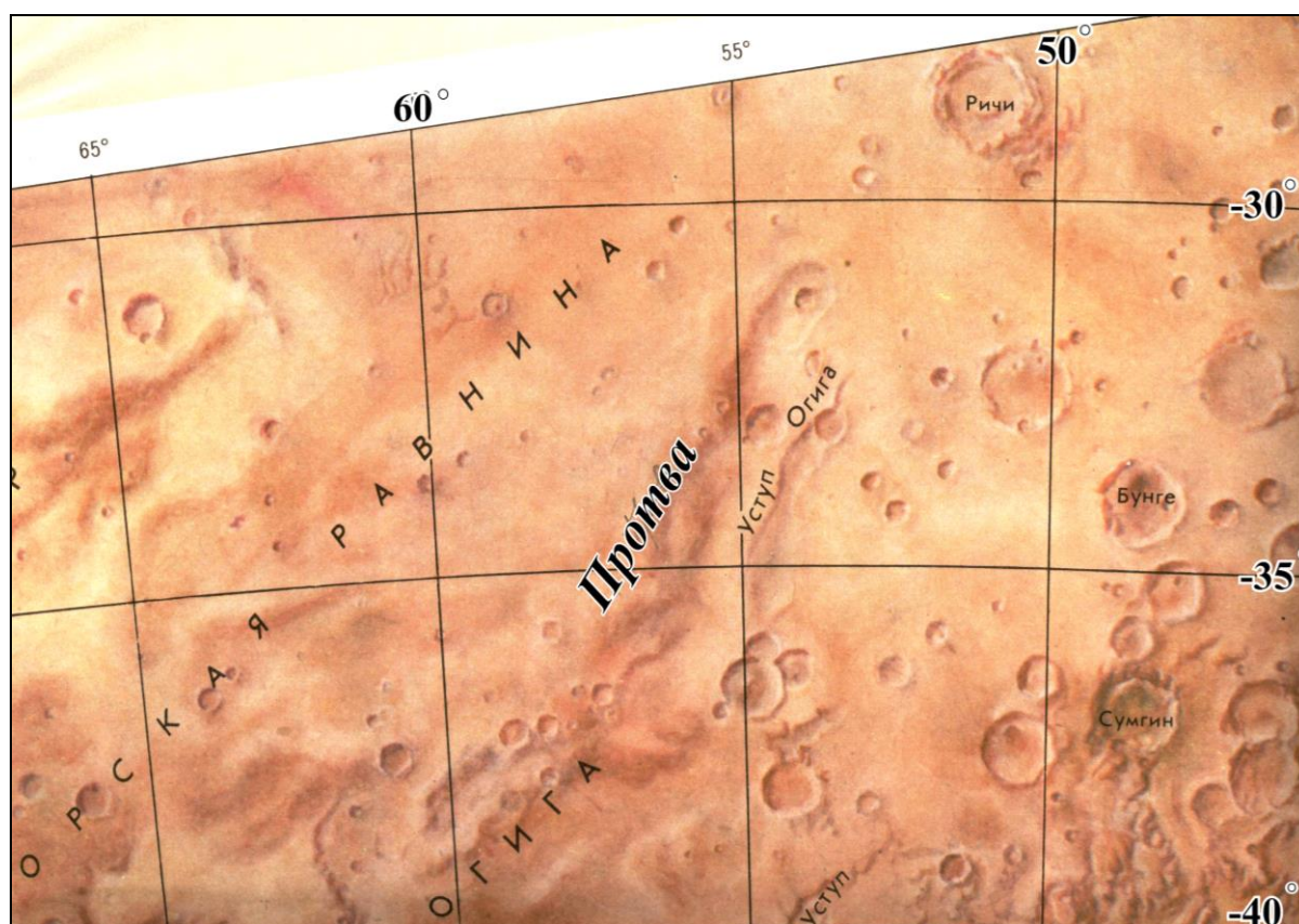
Фрагмент карты поверхности южного полушария Марса. 1977г.
